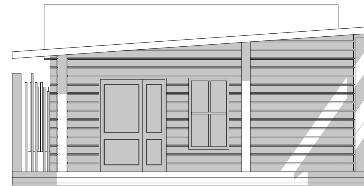
FASAD HUVUDENTRÉ, MOT NORR
