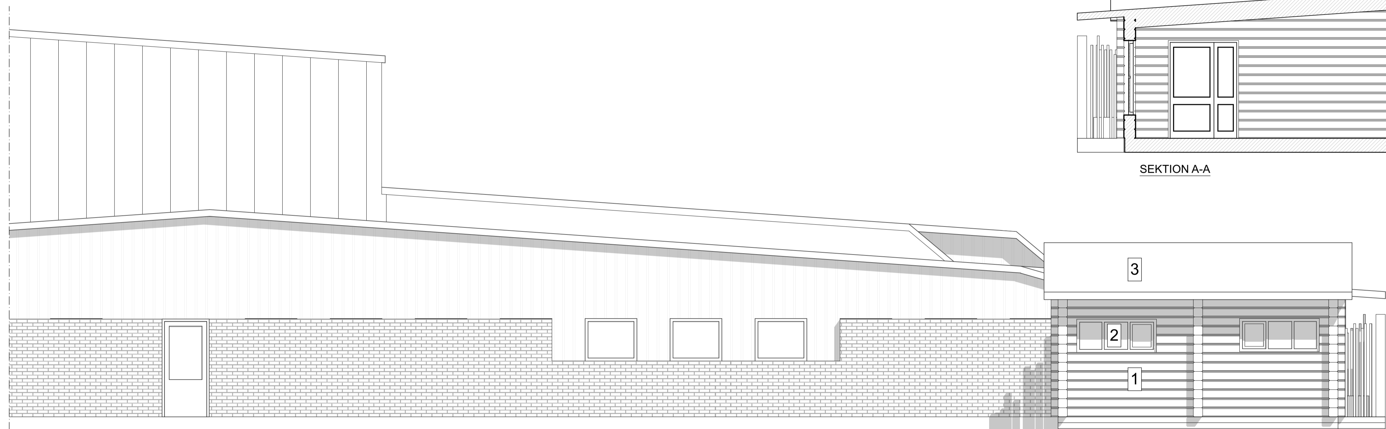
FASAD MOT SÖDER
