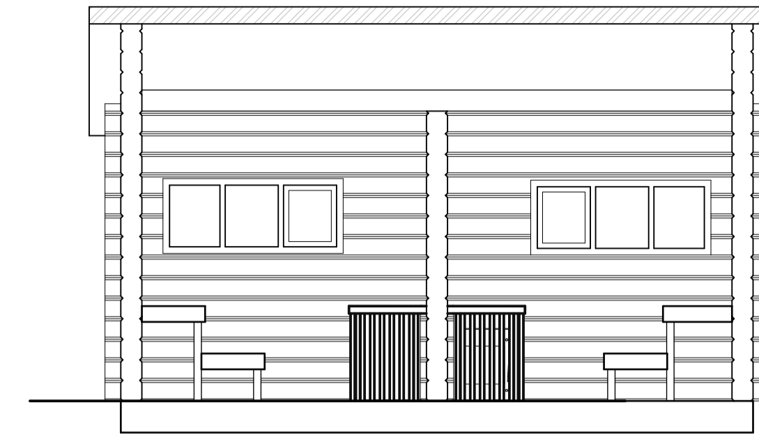
SEKTION B-B
