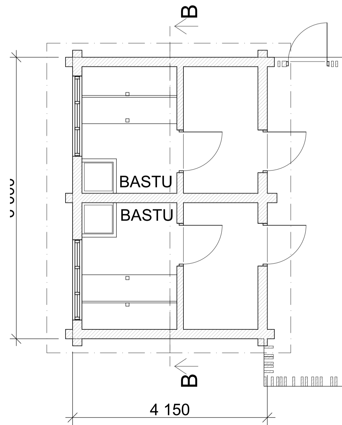
BASTU PLAN
